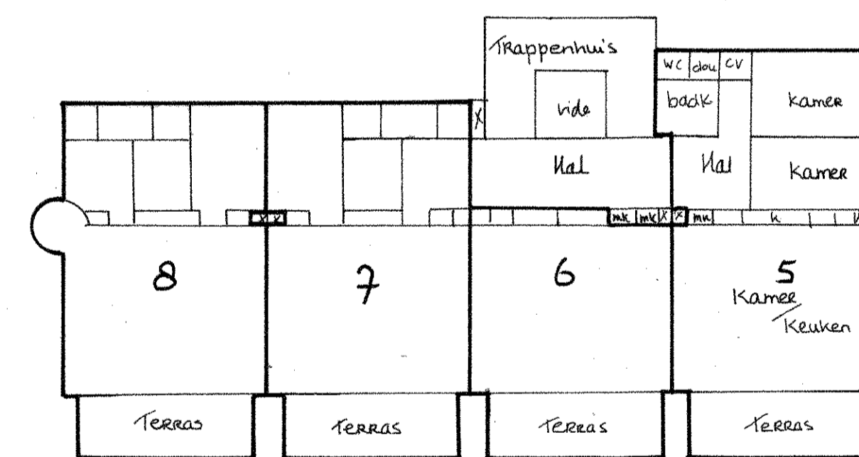
1 e verdieping 1:200
