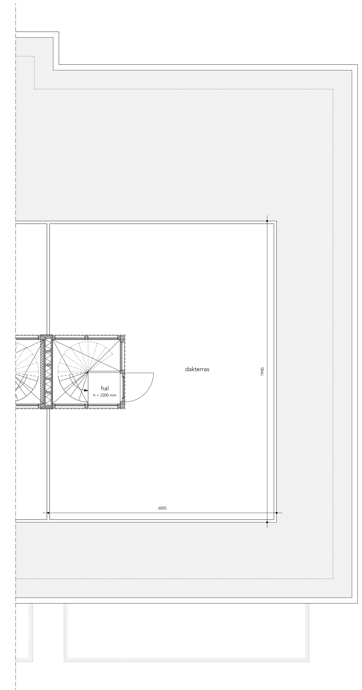
dakopbouw en -terras
