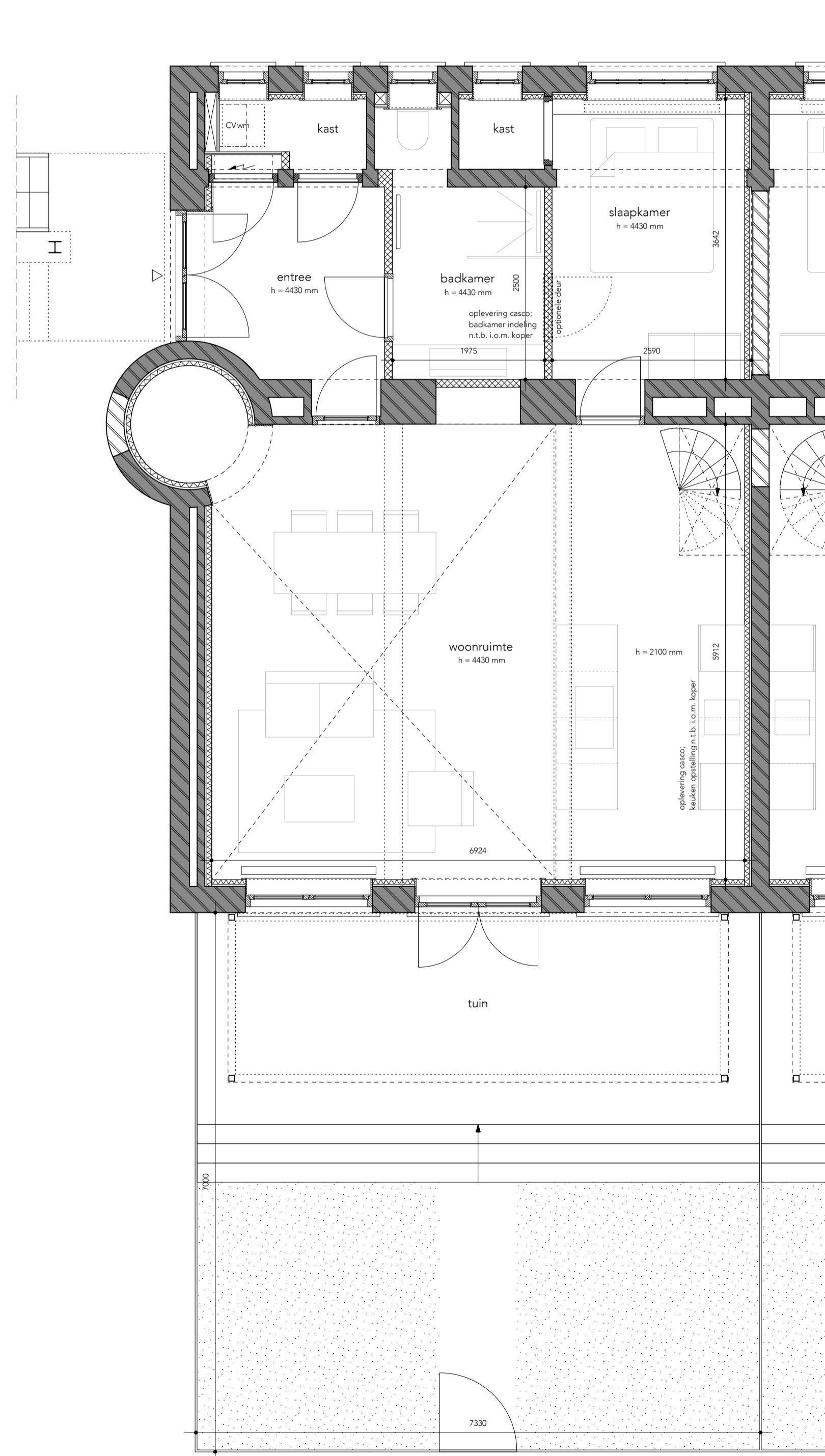
begane grond
