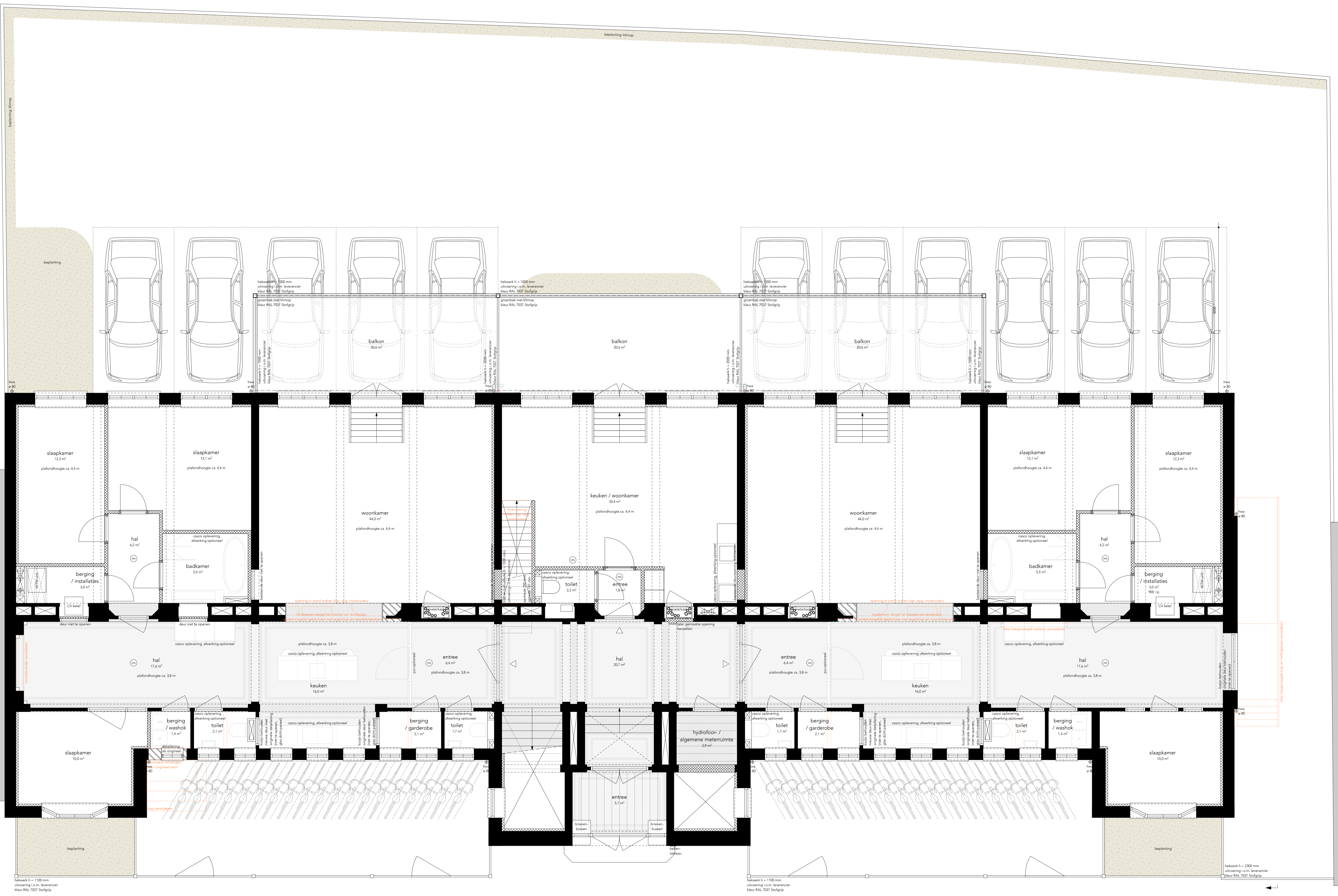
plattegrond bel-etage schaal 1:50 | formaat A1 let op: alle maten zijn circa maten
