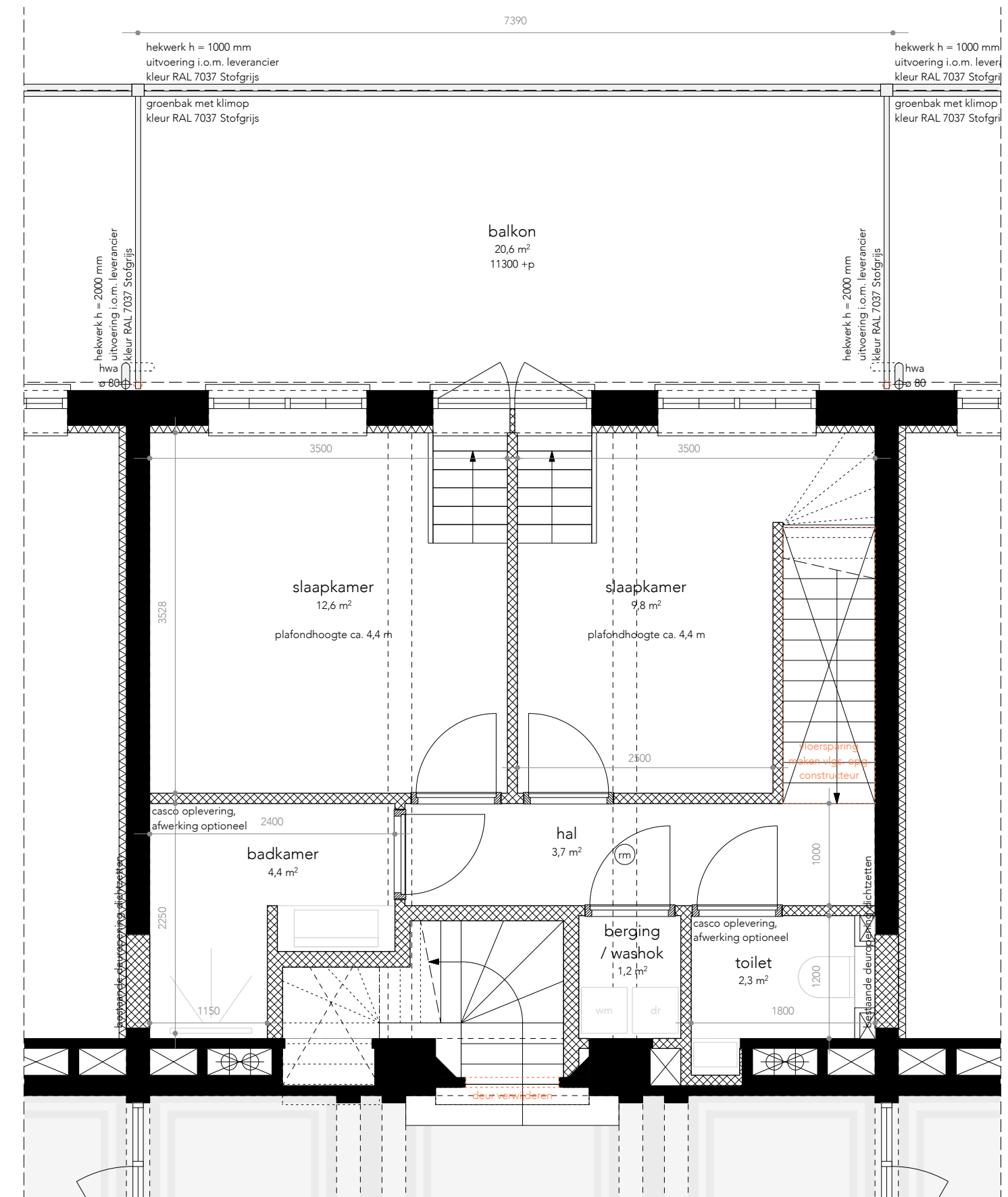
2e verdieping
