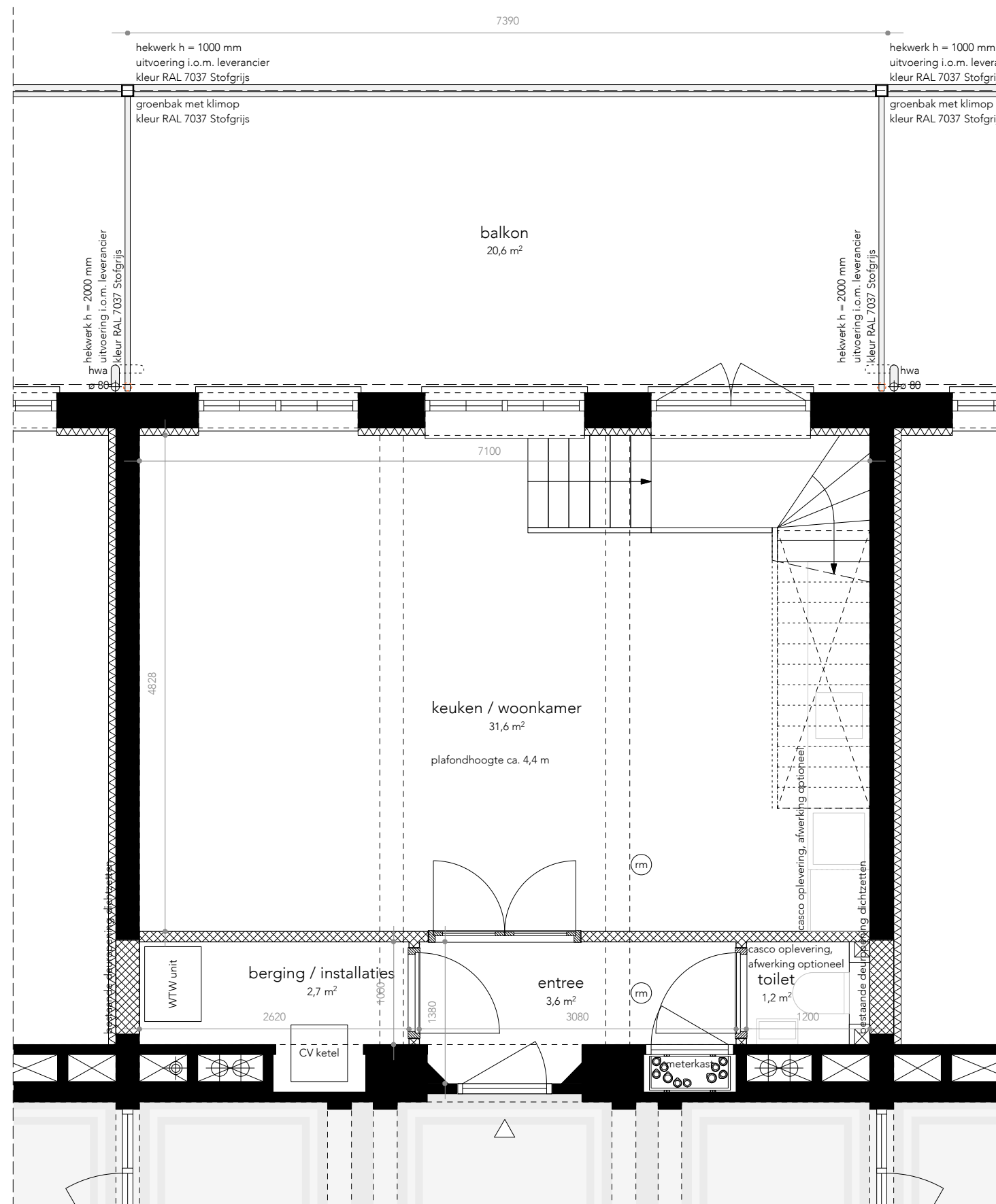
1e verdieping
